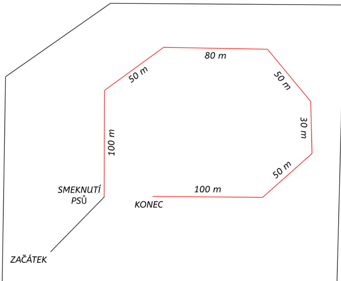
Trať o délce 460 m za použití 6 kladek.
